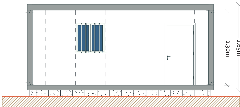
Alzado Frontal
